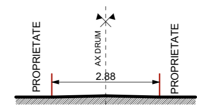
PROFIL A-A SITUATIE EXISTENTA - DE
