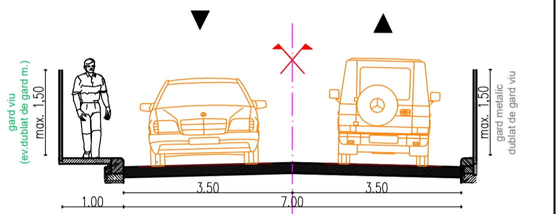
PROFIL TRANSVERSAL STRADA PROPUSA DIN CARE SE FACE ACCESUL PE PROPRIETATI (PARTEA FRONTALA - DE LA INTERSECTIA CU STR. SALISTE)
