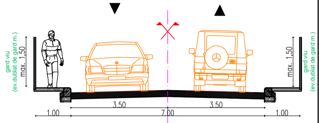
PROFIL TRANSVERSAL STRADA PROPUSA DIN CARE SE FACE ACCESUL PE PROPRIETATI (PARTEA POSTERIOARA)
